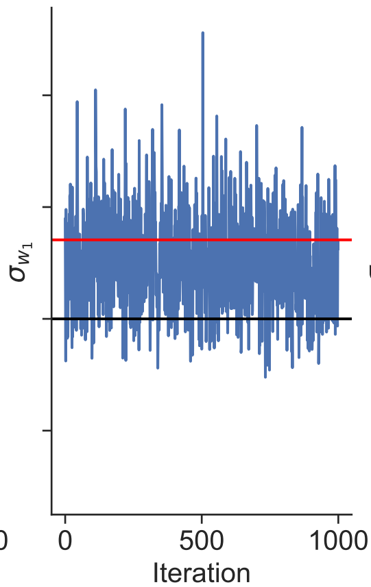
Posterior distributions Dataset 20
